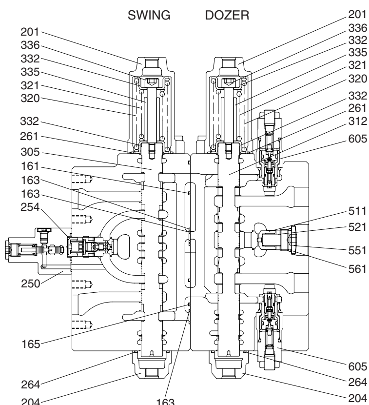
SECTION D-D
