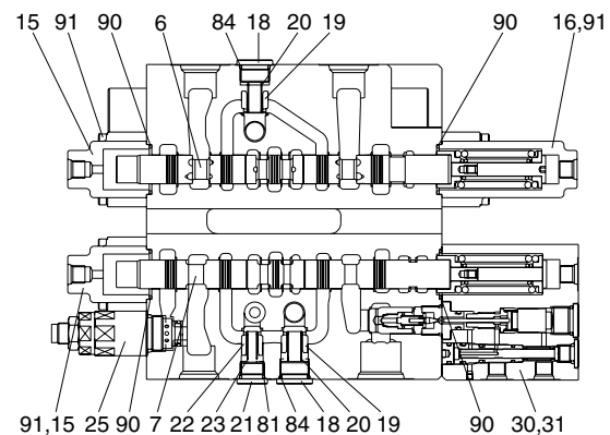
C - C (SWING & BOOM)
