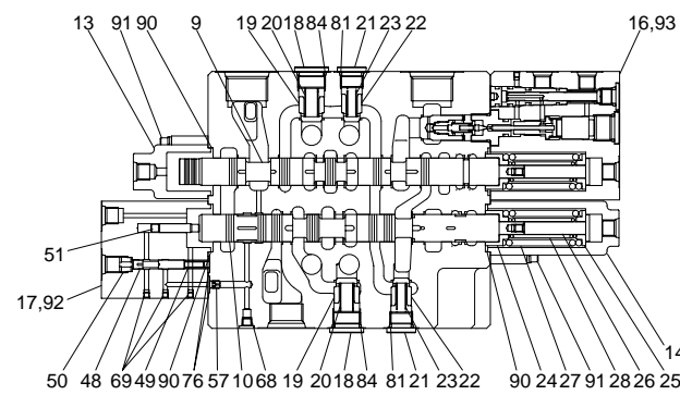
E - E (ARM1 & ARM REGENERATION /BREAKER)
