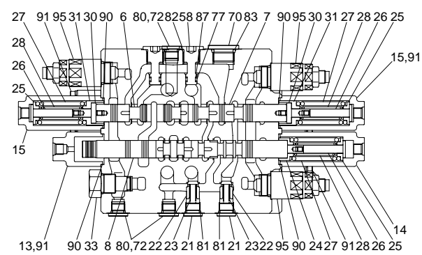
D - D (SWING PRIORITY & BOOM2 & ARM2)
